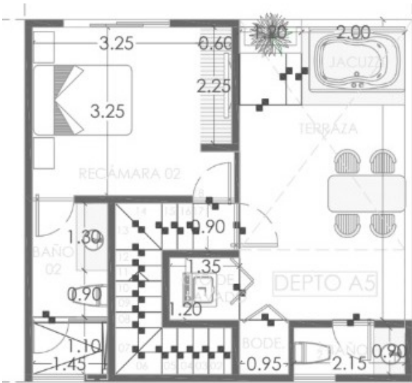
PLANTA ALTA
